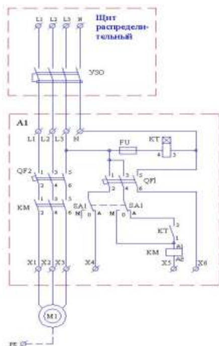
Эл.схема 1
