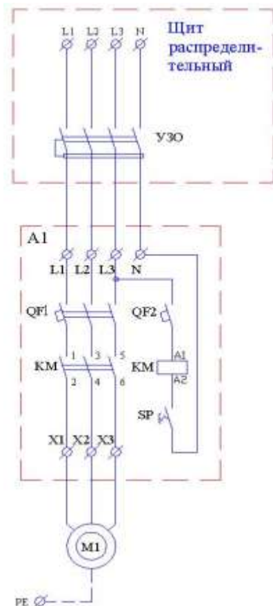
Эл.схема 2
